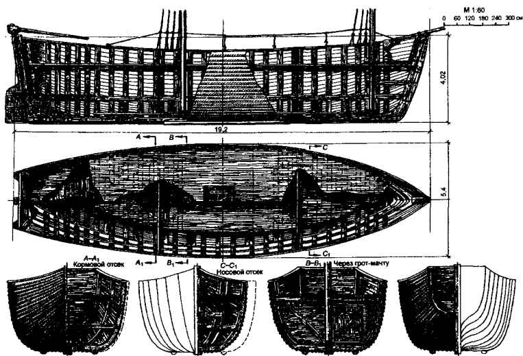
Русский коч, найденный на Груманте.
