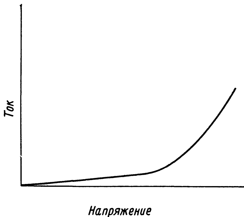
Рис. П.4. Поляризационная кривая.
