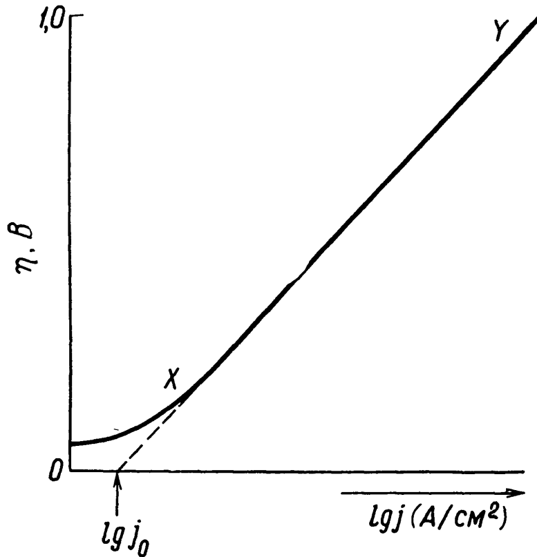
Рис. А.2. Графическое представление уравнения Тафеля.
