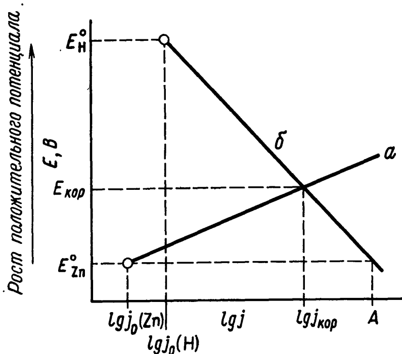
Рис. К.8. Определение потенциалов коррозии.
