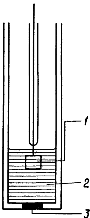
Рис. И. 1. Твердотельный ионоселективный электрод.
