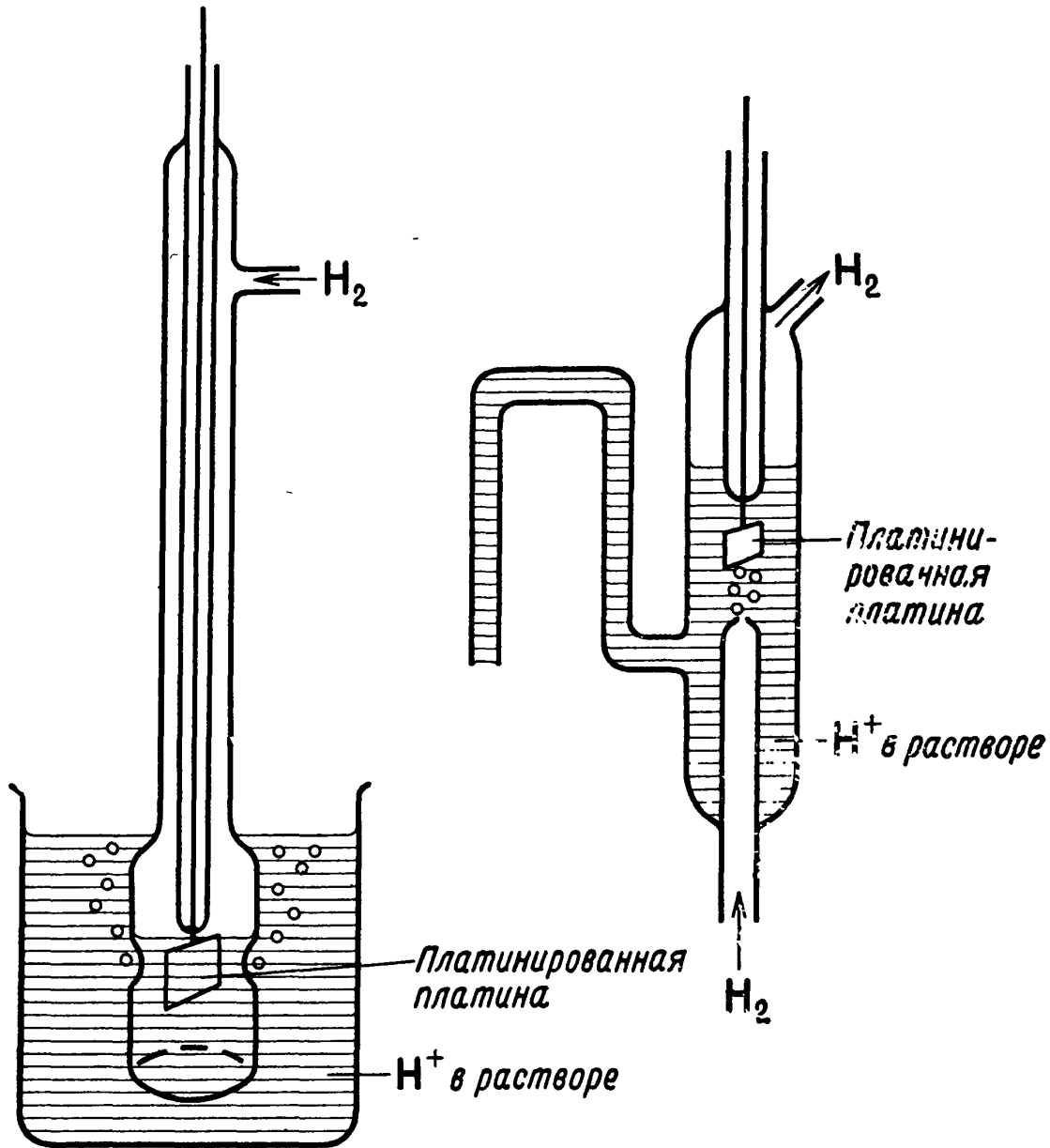
Рис. В.1. Типичные формы водородного электрода.
