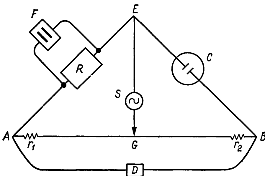
Рис. Э.8. Мост для измерения электропроводности.
