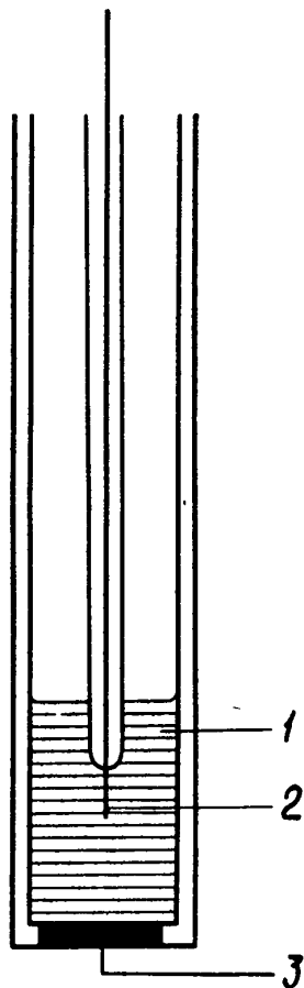
Рис. И. 2. Ионоселективный электрод с гетерогенной мембраной.
