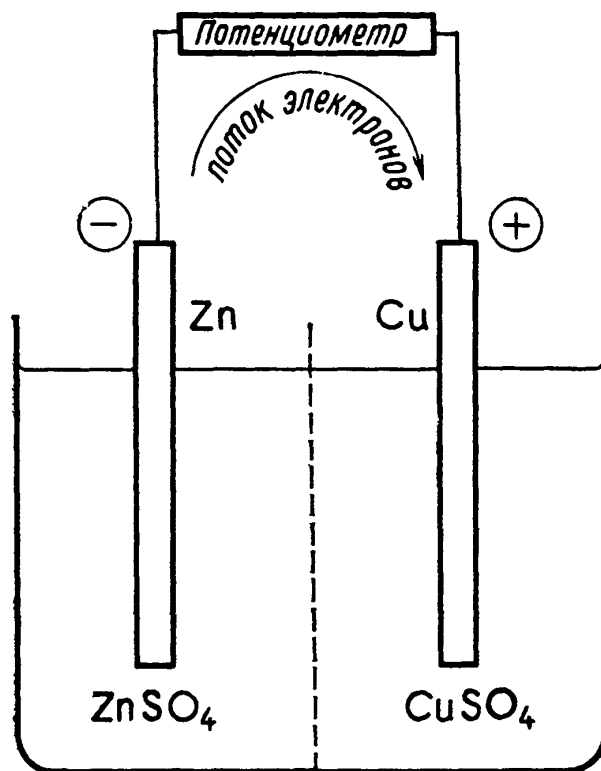
Рис. Э.16. Схема элемента Даниэля.
