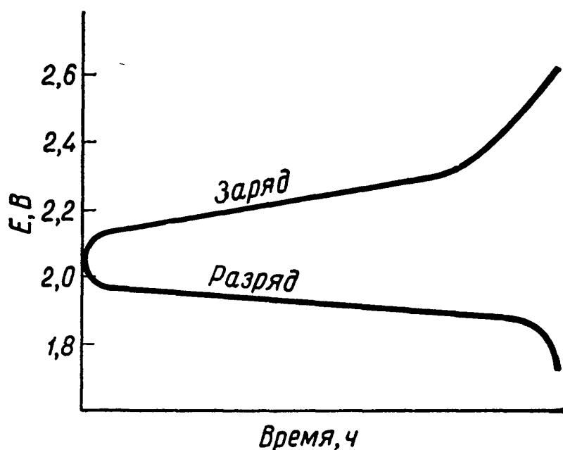
Рис. А. 1. Кривые заряда и разряда для свинцового аккумулятора.
