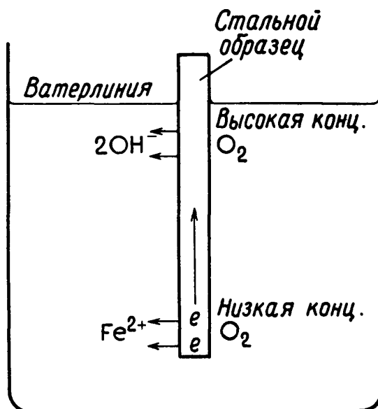
Рис. К.6. Коррозия металла в глубине раствора.
