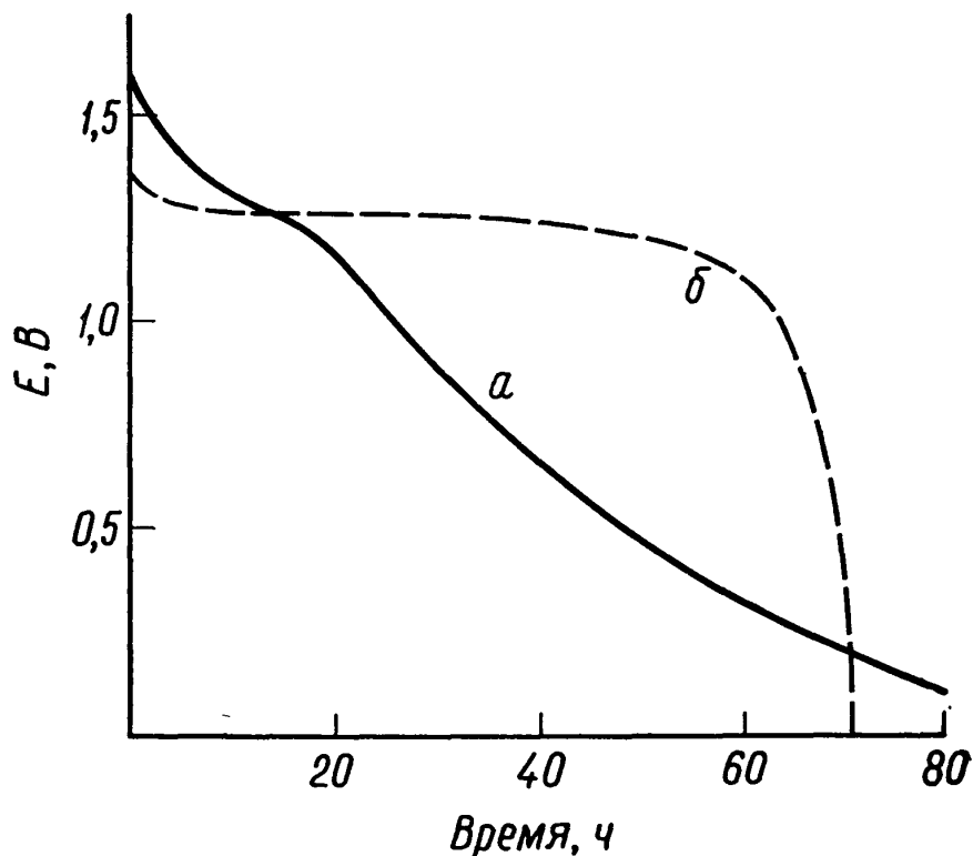
Рис. П.3. Разрядные кривые.
