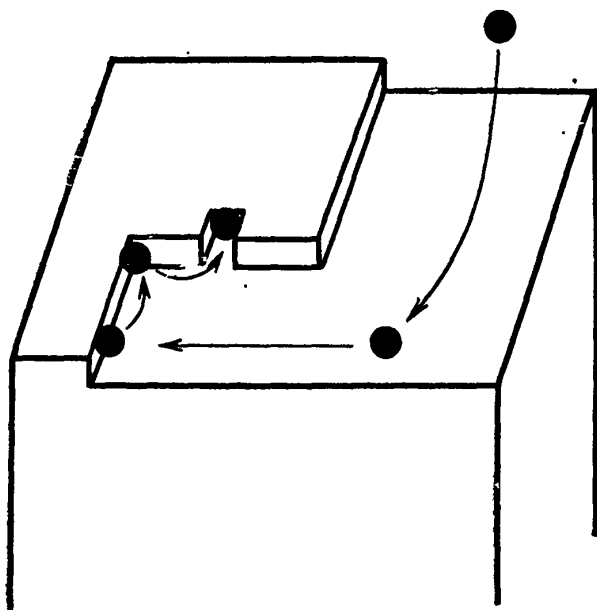
Рис. Э.5. Стадии процесса осаждения иона металла.
