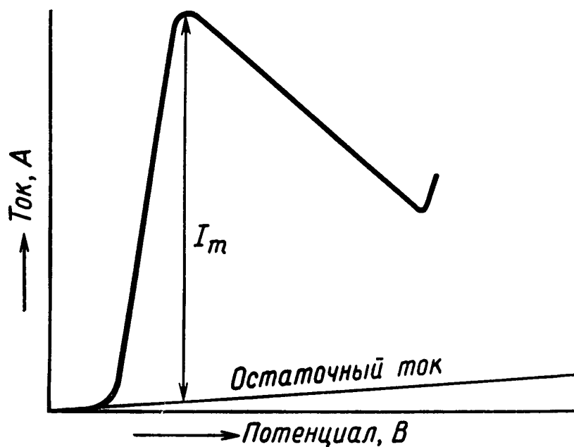
Рис. X.1. Хроноамперометрическая кривая при линейной развертке потенциала.
