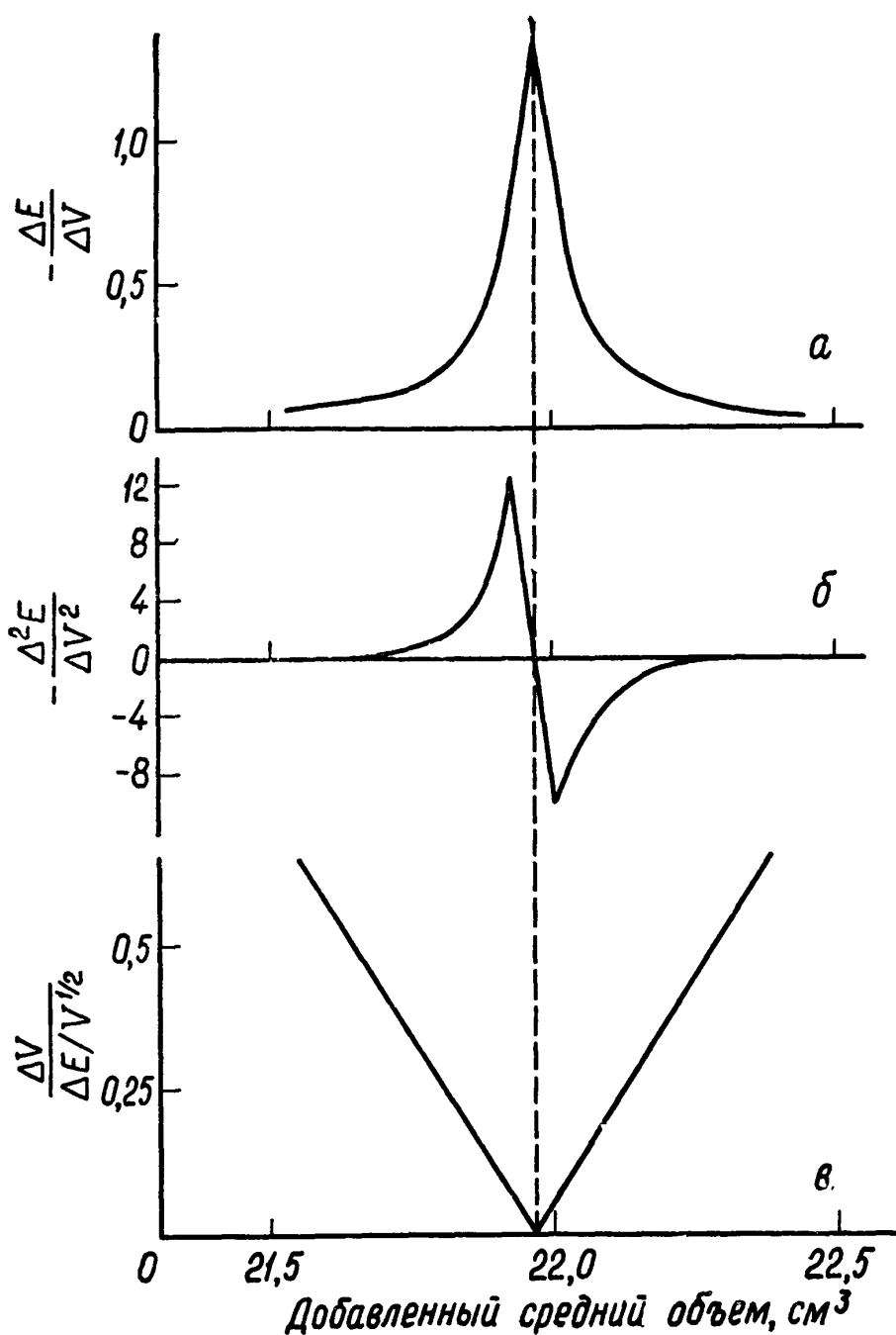
Рис. П.11. Дифференциальные кривые титрования.
