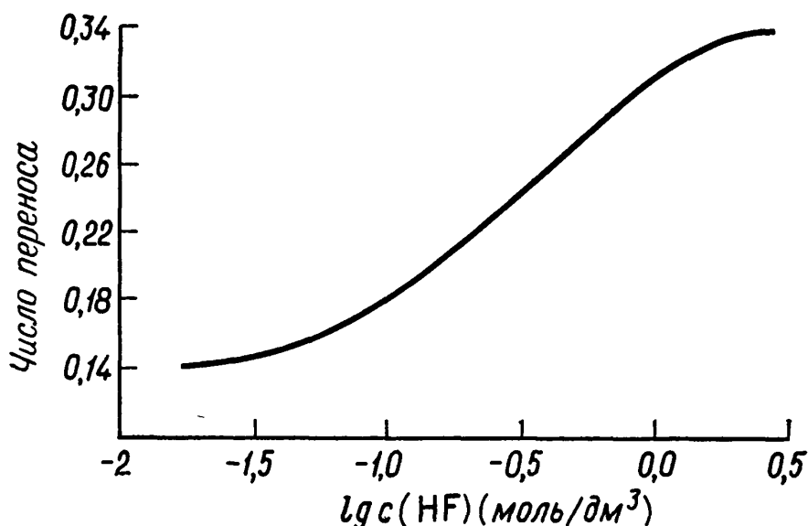
Рис. Ч. 1. Кажущиеся числа переноса анионов для растворов HF при 298 К.
