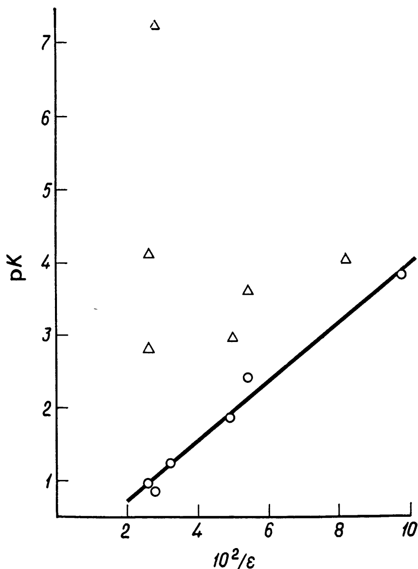
Рис. Н.1. Значения pK в неводных растворителях: \bigcirc пикрат тетраэтиламмония; \triangle пикрат лития.
