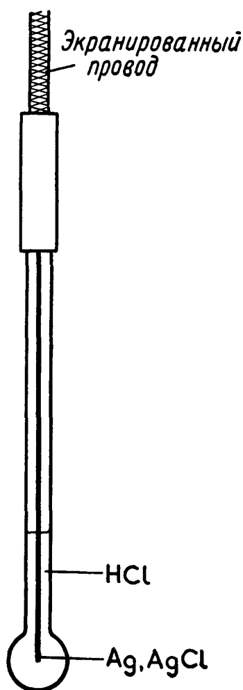
Рис. С.2. Стеклянный электрод.
