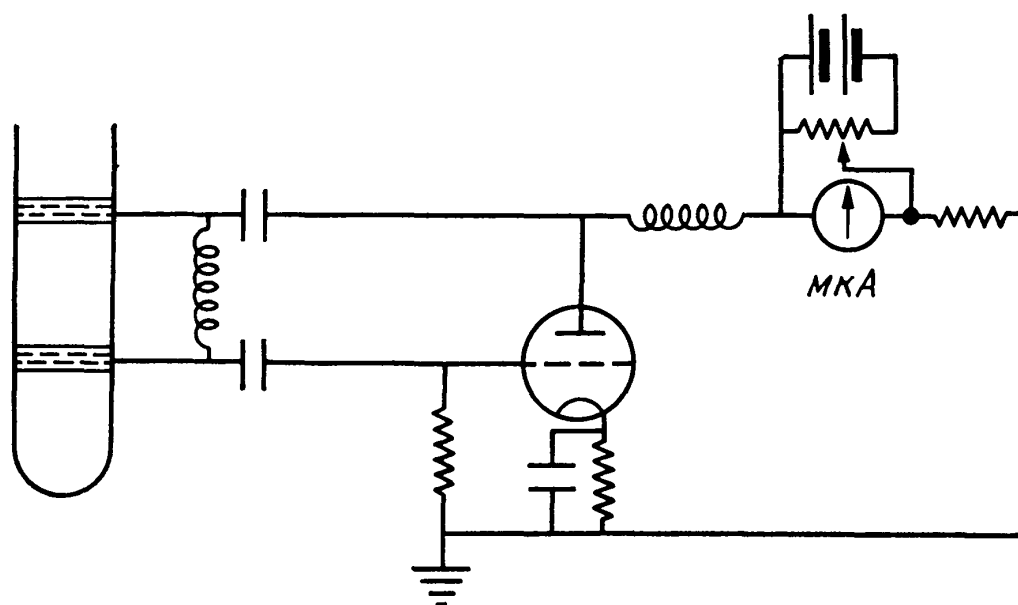
Рис. О.7. Схема простого осциллометра.
