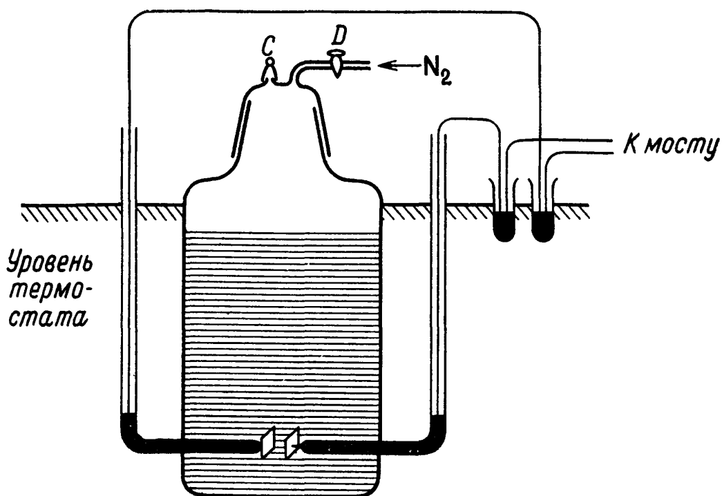
Рис. Э.9. Ячейка для измерения электропроводности разбавленных растворов.
