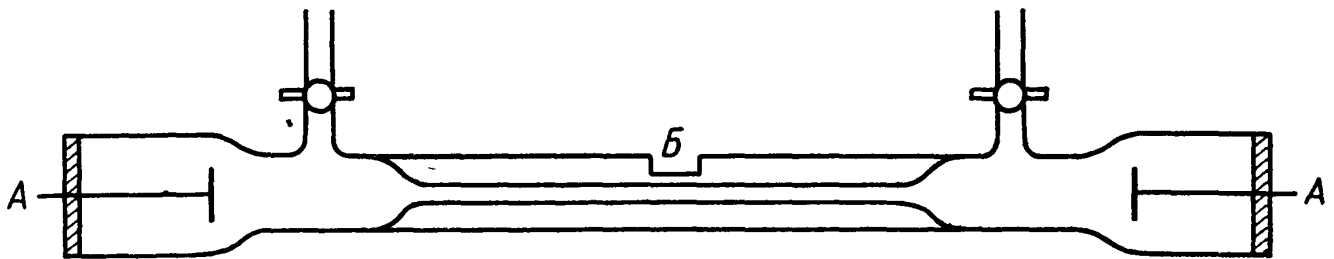
Рис. Э. 14. Микроячейка для проведения электрофореза.
