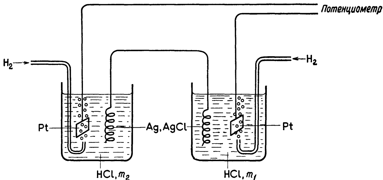
Рис. К.5. Схема концентрационной цепи.
