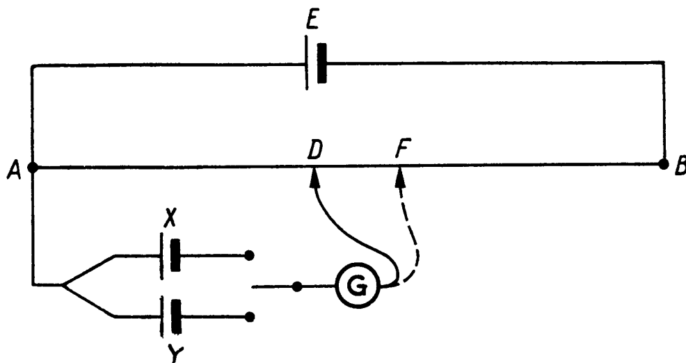
Рис. П.9. Принципиальная схема проволоочного потенциометра.
