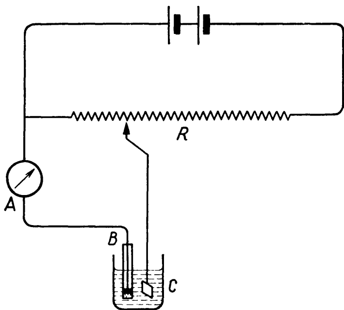
Рис. А.3. Схема установки для амперометрического титрования.
