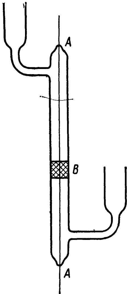
Рис. П.8. Ячейка для измерения потенциала течения.
