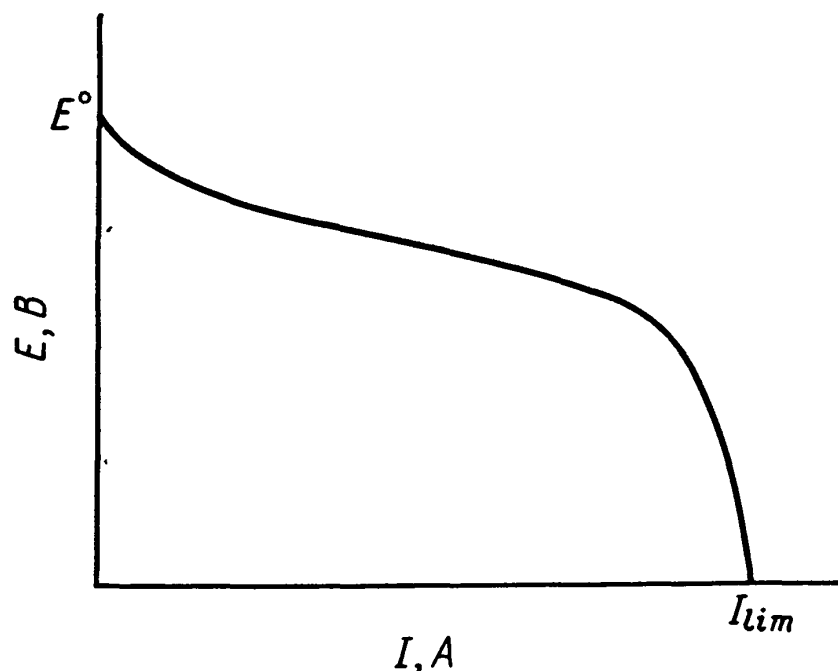
Рис. П.2. Типичная вольт-амперная кривая.
