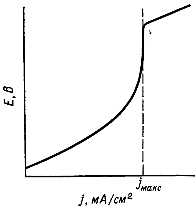
Рис. П.20. Зависимость потенциала — плотность тока при наличии концентрационного перенапряжения.
