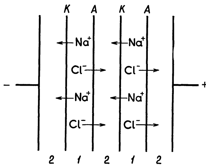
Рис. О.6. Схема электролизера для опреснения воды.
