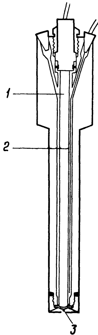
Рис. Д.1 Датчик аммиака.
