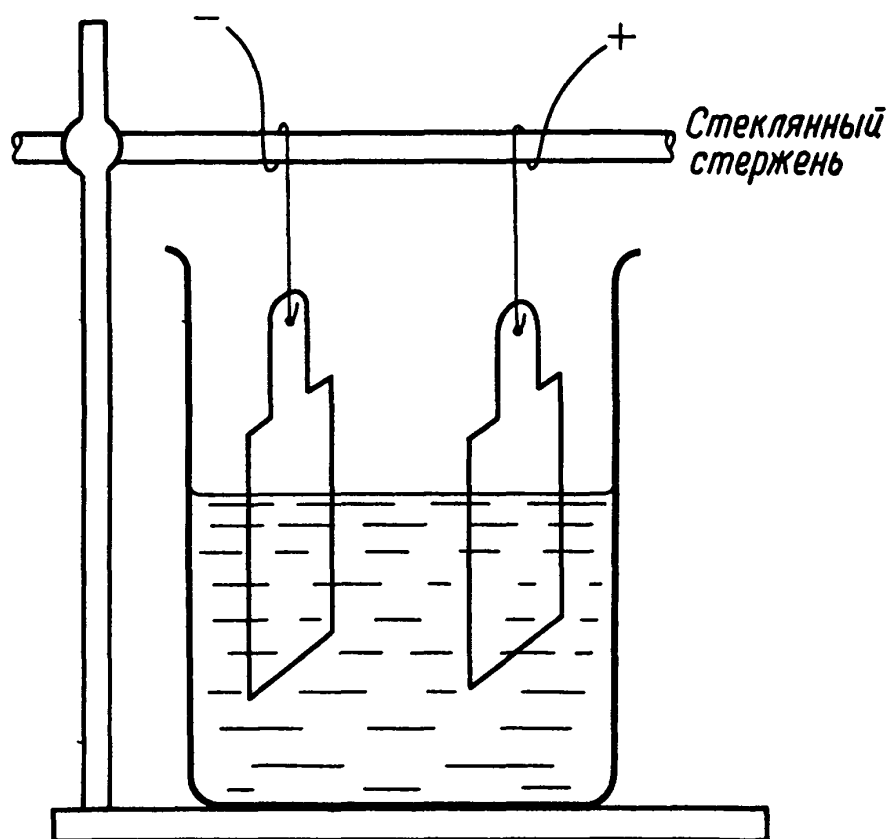
Рис. М. 1. Медный кулонометр для небольших токов.
