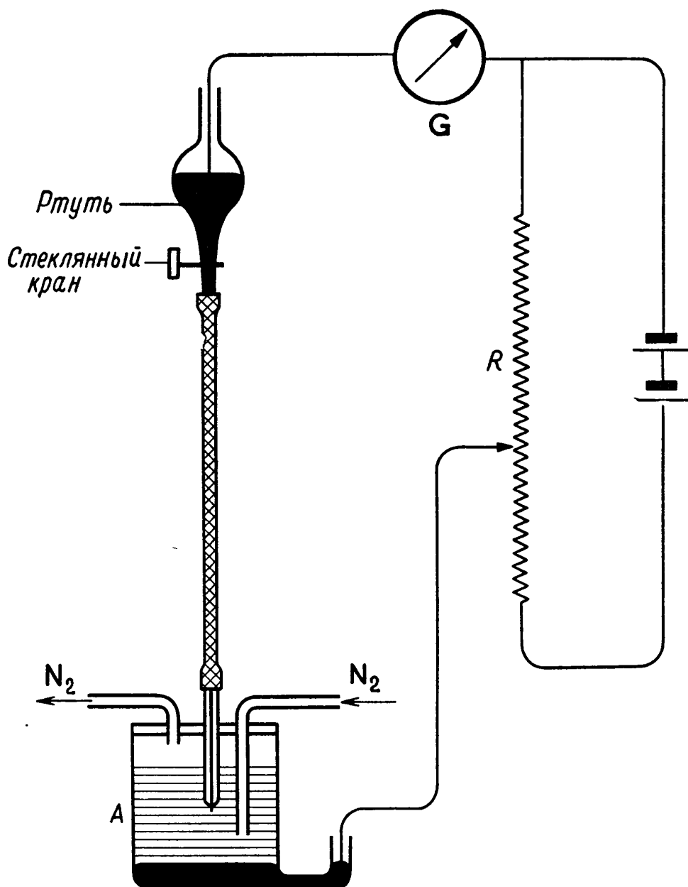
Рис. П.6. Принципиальная схема полярографа.
