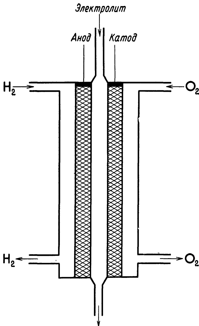
Рис. Т.4. Схема водородно-кислородного топливного элемента
