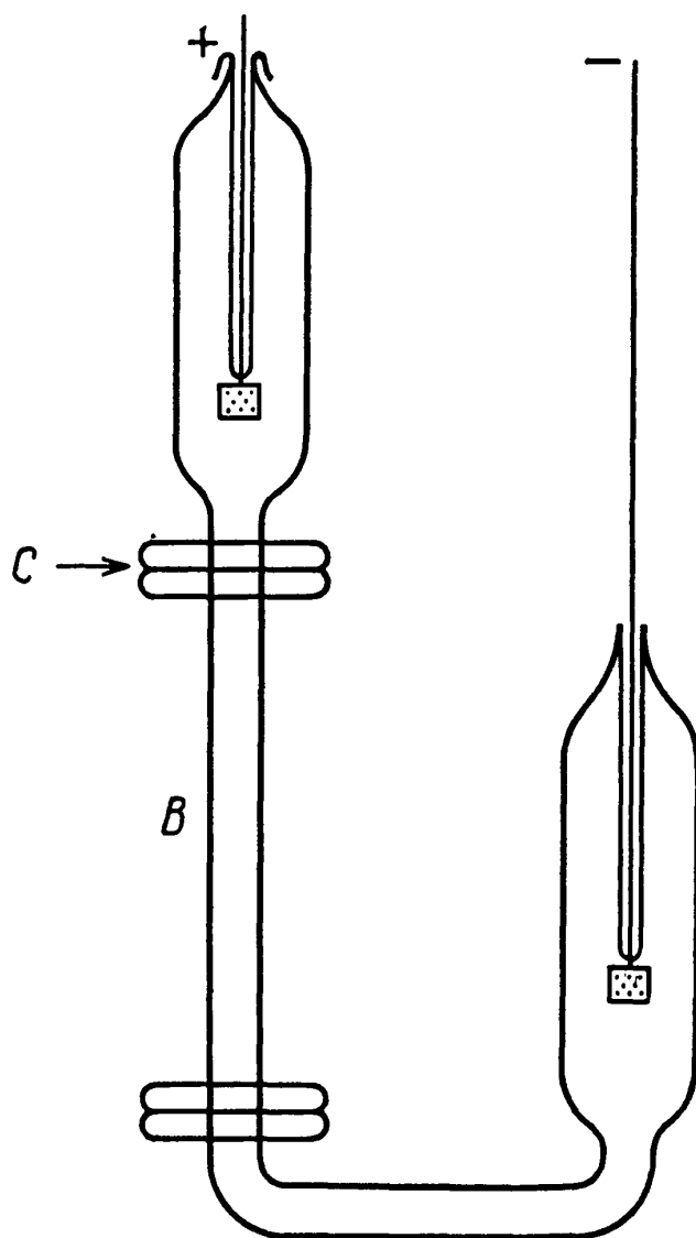
Рис. М.5. Прибор для проведения измерений методом движущейся границы.
