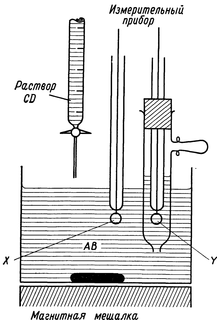
Рис. П. 16. Прибор для проведения дифференциального титрования.
