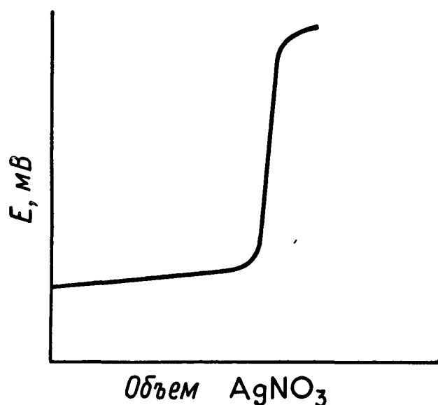
Рис. П.13. Кривая осадительного титрования.
