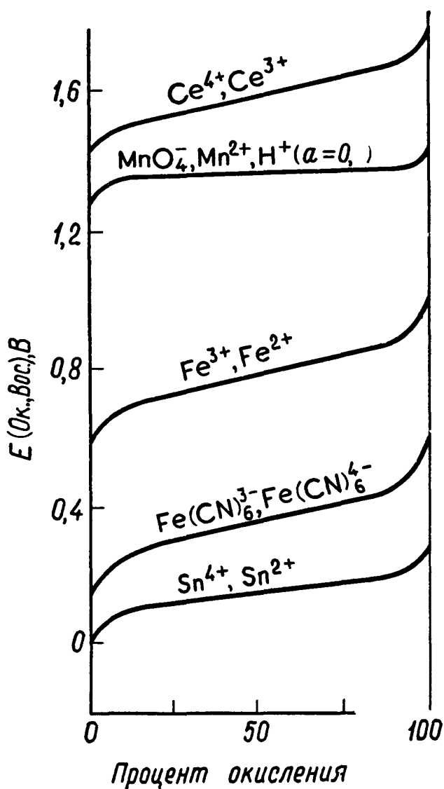
Рис. O.2. Окислительно-восстановительные потенциалы.
