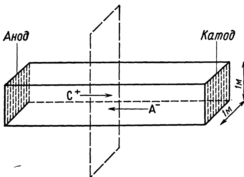
Рис. Э. 7. Диаграмма, поясняющая проводимость электролита.
