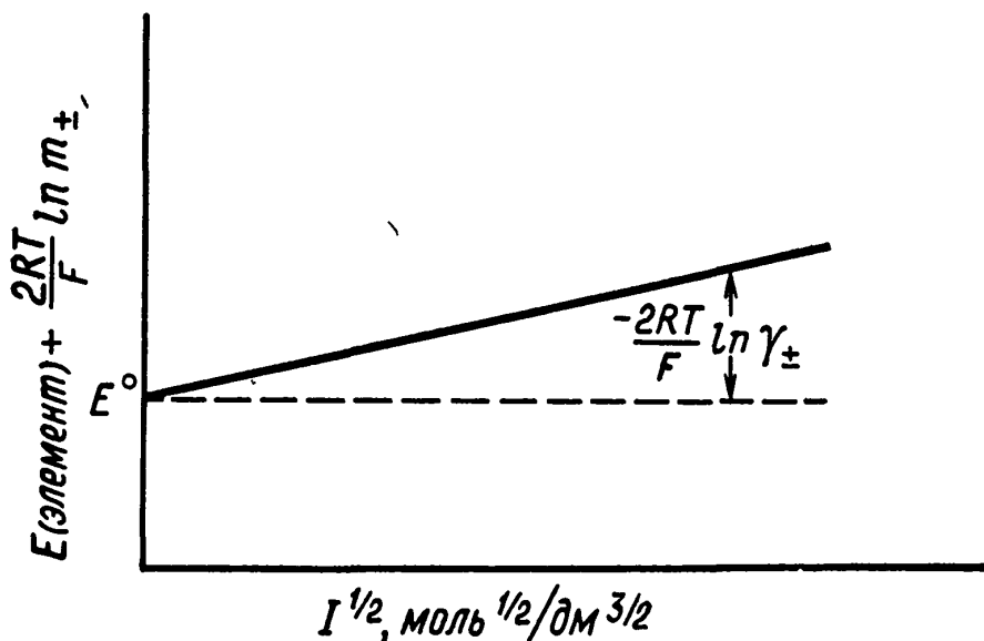
Рис. Э. 1. Графическое определение величины E^\circ (элемент).
