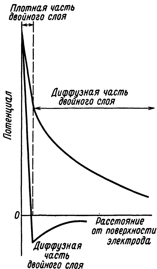
Рис. Д.3. Распределение потенциала в двойном слое по Штерну.
