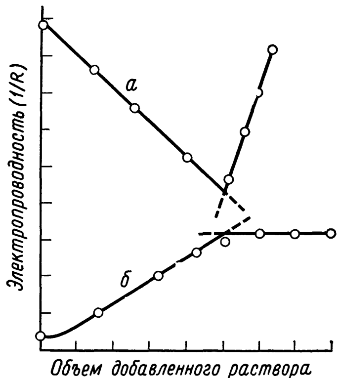
Рис. К. 3. Кондуктометрические кривые титрования.
