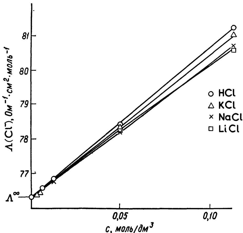
Рис. М.9. Ионная электропроводность растворов, содержащих хлорид-ион.
