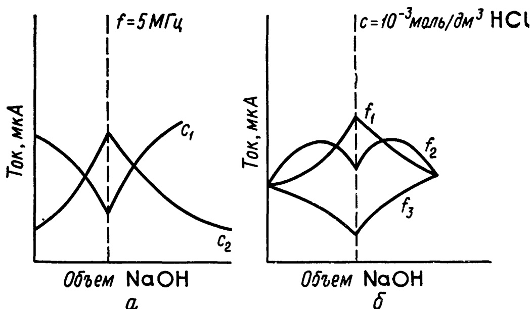
Рис. О.8. Типичные кривые титрования.
