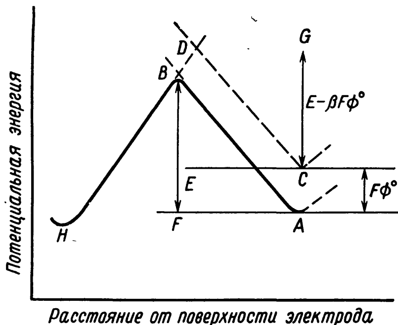
Рис. М.6. Кривая потенциальной энергии.
