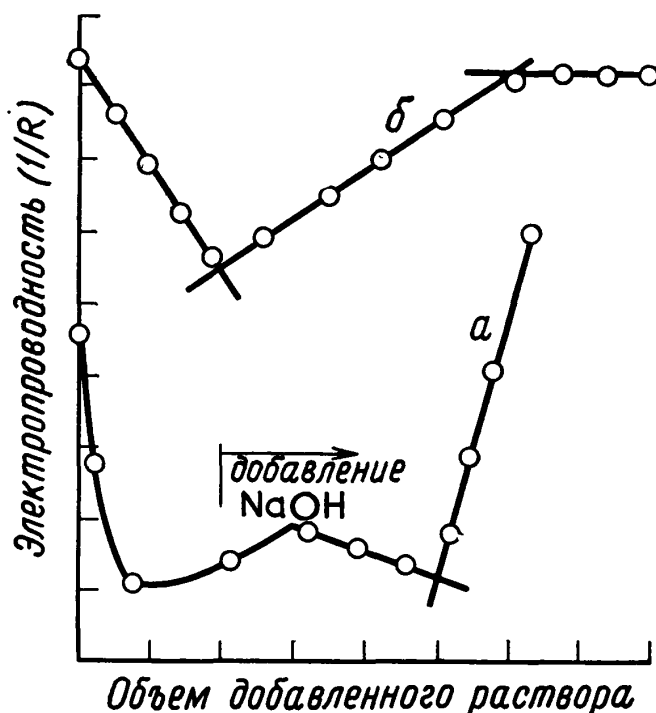
Рис. К. 4. Кондуктометрические кривые титрования.
