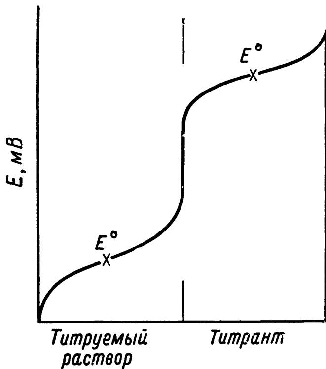
Рис. П.15. Кривая окислительно-восстановительного титрования.
