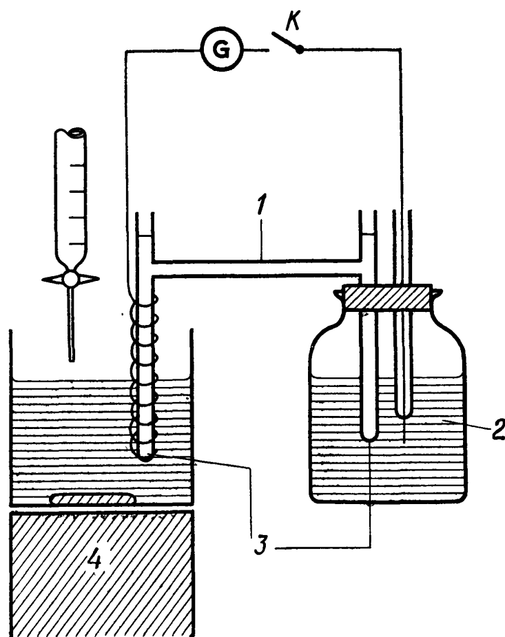
Рис. П.17. Прибор для проведения титрования по методу конечной точки.
