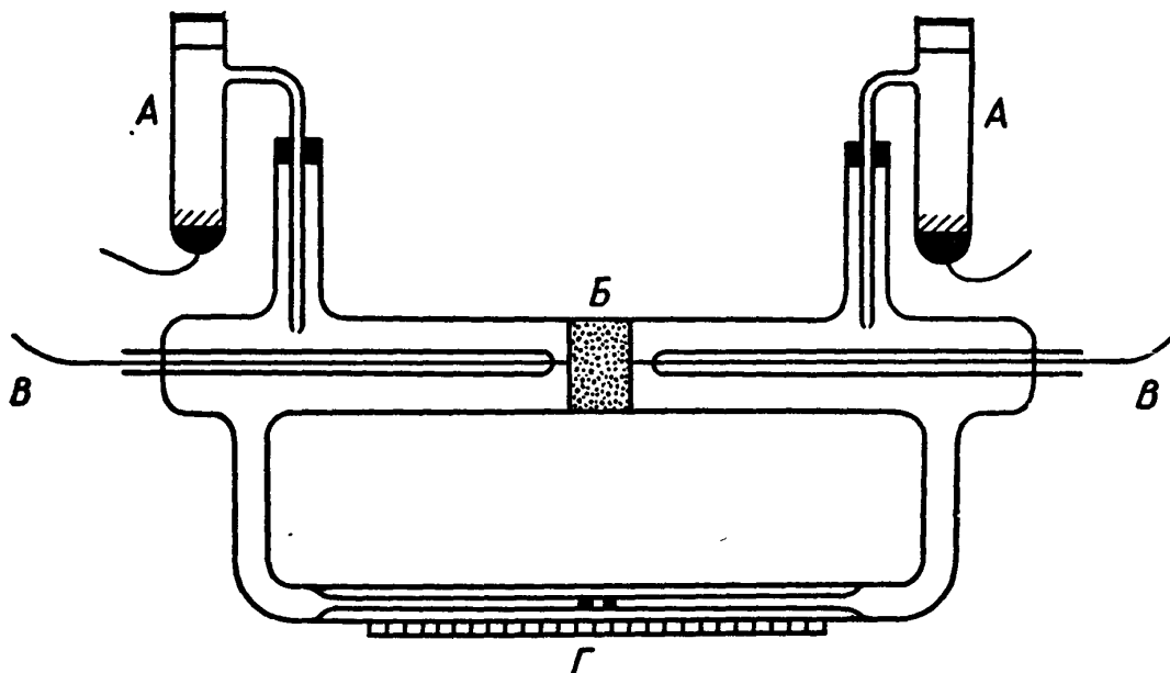
Рис. Э.6. Электроосмотическая ячейка.
