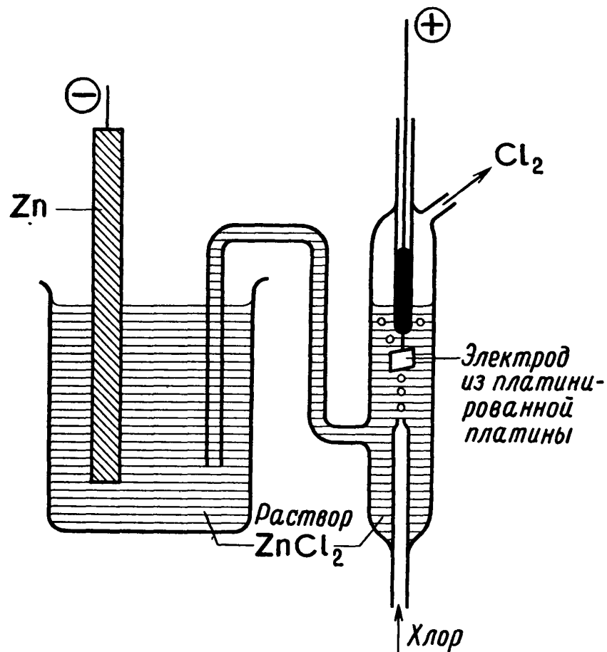
Рис. O.1. Типичный цинк-хлорный элемент.
